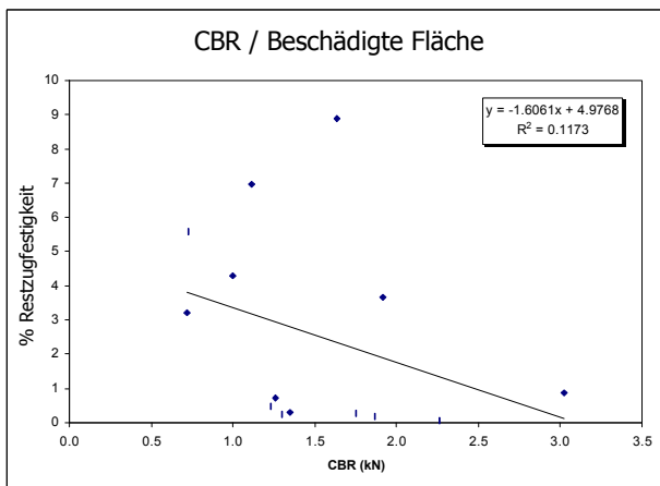
Bild 8: Korrelation zwischen CBR und beschädigter Fläche.
