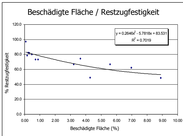
Bild 3: Korrelation zwischen beschädigter Fläche und Restfestigkeit.
