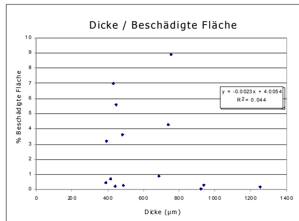
Bild 5: Korrelation zwischen Dicke und beschädigter Fläche.
