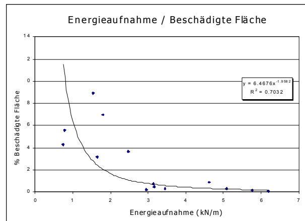
Bild 11: Korrelation zwischen Energieaufnahme und beschädigter Fläche.
