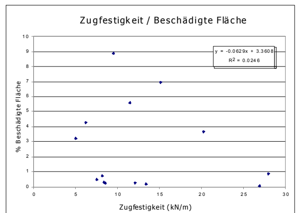
Bild 6: Korrelation zwischen Zugfestigkeit und beschädigter Fläche.
