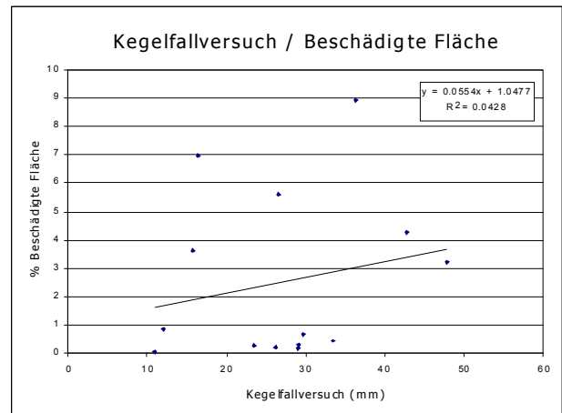
Bild 10: Korrelation zwischen Kegelfallversuch und beschädigter Fläche.
