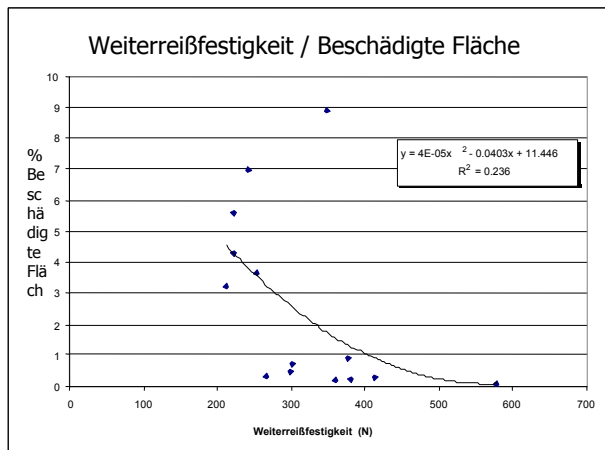
Bild 9: Korrelation zwischen Weiterreißfestigkeit und beschädigter Fläche.
