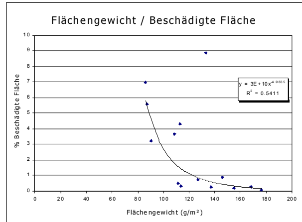
Bild 4: Korrelation zwischen Flächengewicht und beschädigter Fläche.
