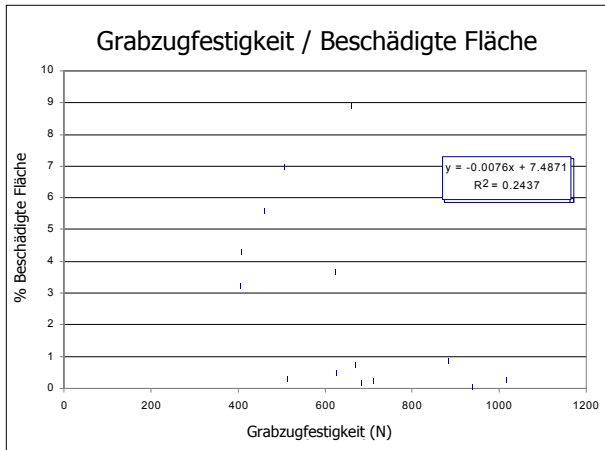
Bild 7: Korrelation zwischen Grabzugfestigkeit und beschädigter Fläche.
